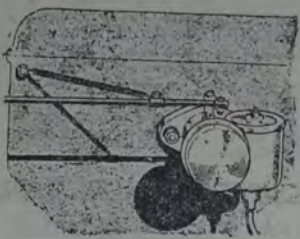
Fig. 1. — El control del acelerador es difícil cuando el resorte es demasiado débil.
