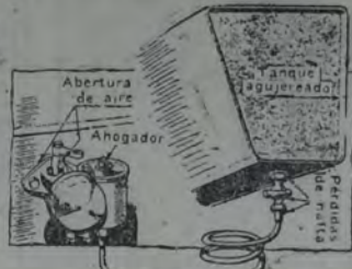
Fig. 2. — La pérdida de nafta por juntas y uniones causa un aumento directo en el consumo de combustible y la entrada adicional de aire empobrece la mezcla combustible.
